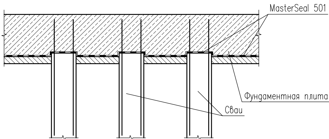
Гидроизоляция снизу плитного фундамента на свайном основании
